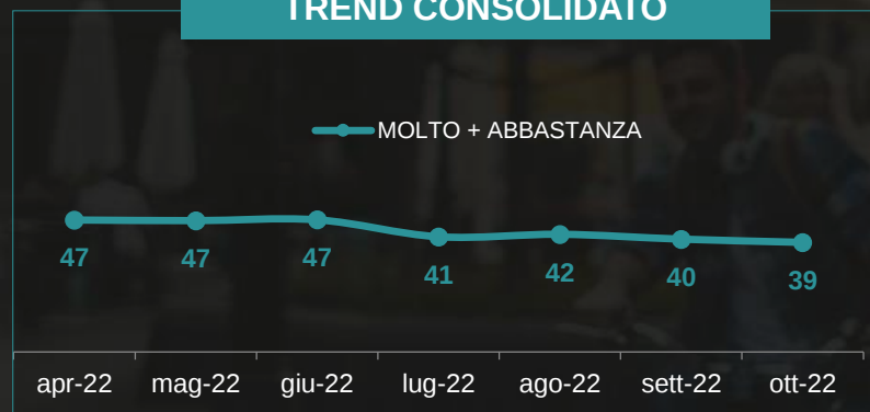
TREND CONSOLIDATO
